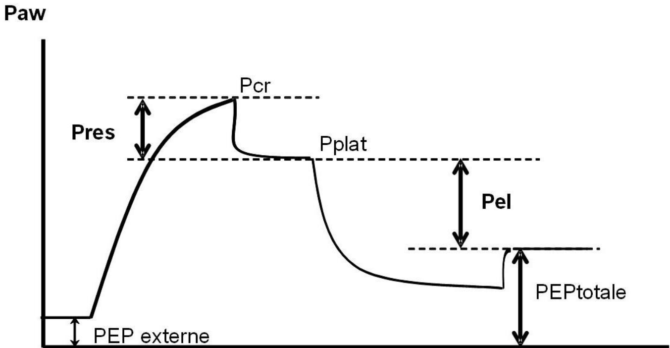
Courbe de pression en présence d'une PEP intrinsèque
