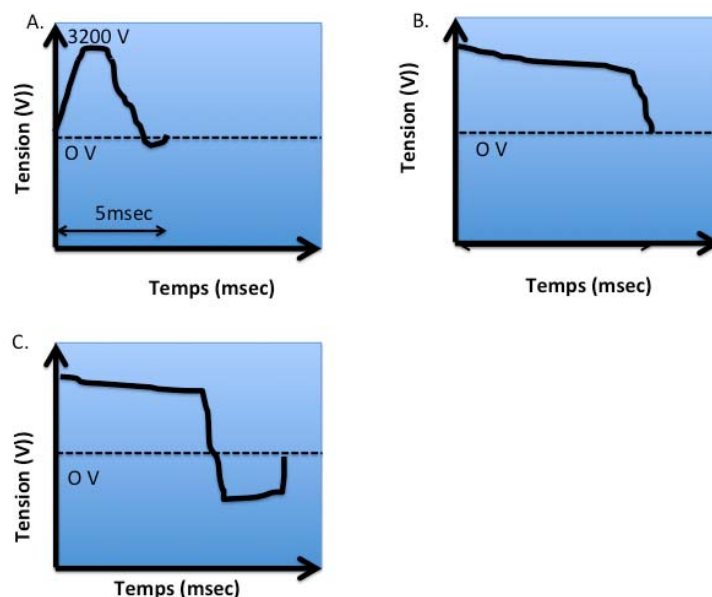
Figure 1. Formes d'ondes électriques de défibrillation. A. Onde monophasique sinusoïdale amortie ; B. Onde monophasique exponentielle tronquée ; C. Onde biphasique exponentielle
