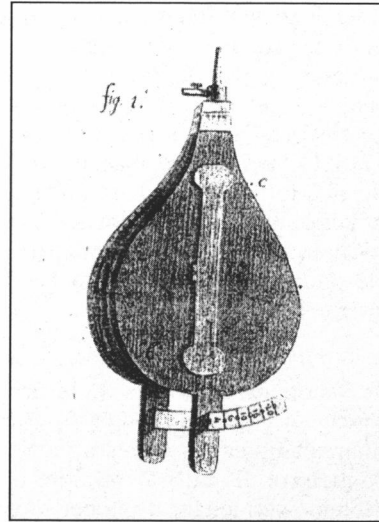
Fig. 2 : Soufflet calibré de J. Leroy d'Etiolles en 1827 [32].
